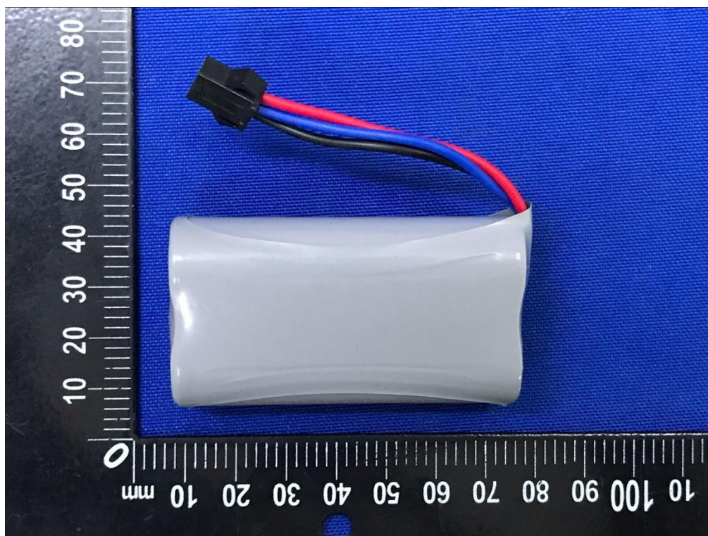
电池反面
